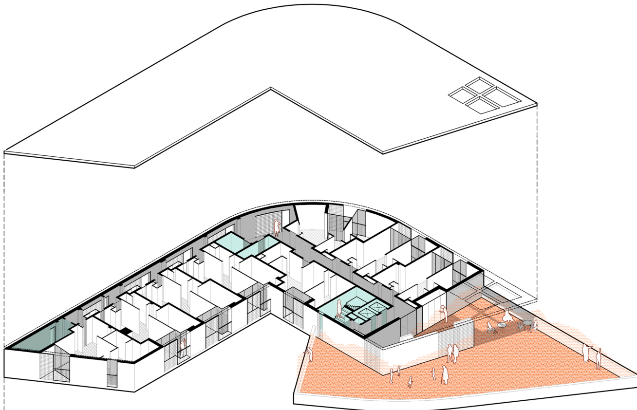
planta 3 _+166,90
