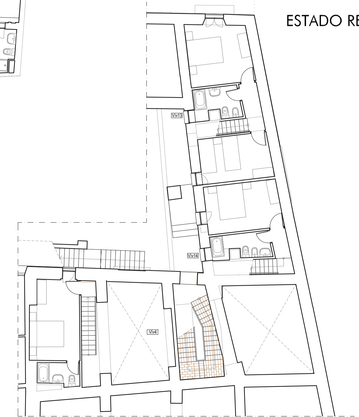
ESTADO REFORMADO_ENTREPLANTA 1/150
