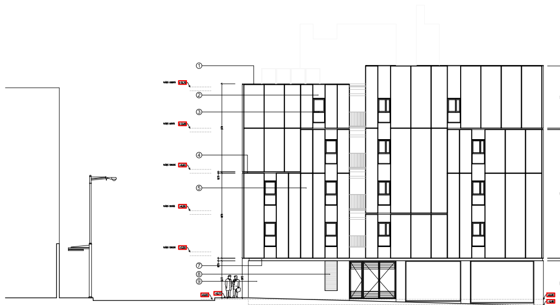
FAÇANA NORD B-B' A1-1/100 A3-1/200
