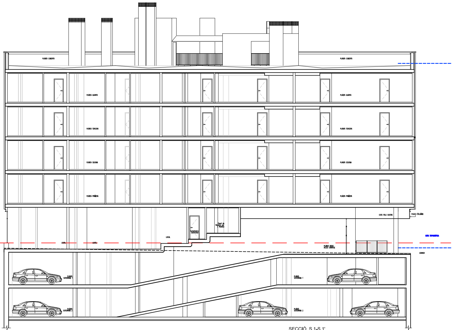
SECCIÓ S.1-S.1' E=1/100
