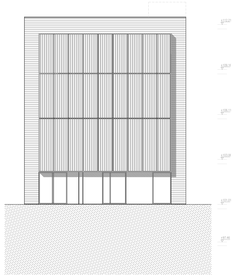
FAÇANA INTERIOR E: 1/50 A-3: E: 1/100
