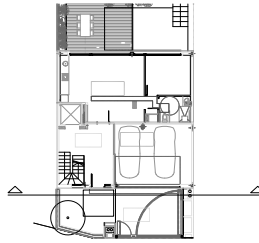
PLANTA ESQUEMÀTICA. E 1/200-A1
