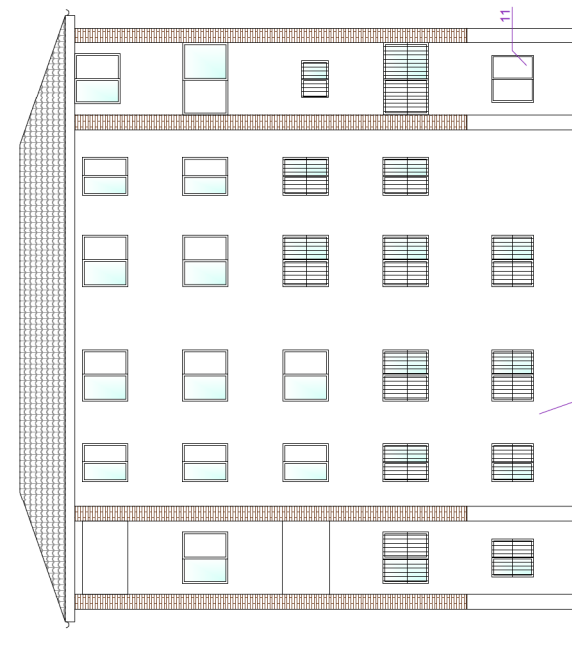
ALZADO PASO PARA ANGELES ARROYO CASTRO
