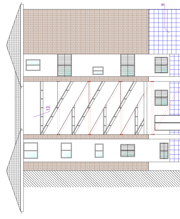
ALZADO OESTE
