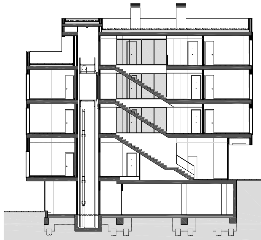
0 3 Secció B
