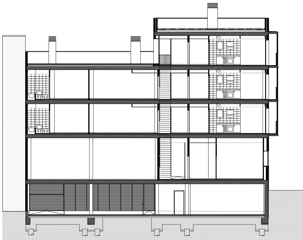
Secció A
