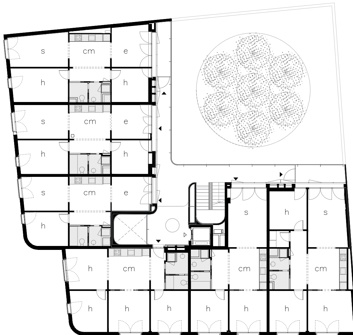
PLANTA TIPO
