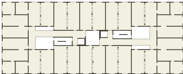
PLANTA TIPO
