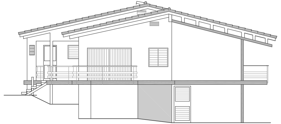
FAÇANA PONENT. ESTAT INICIAL
