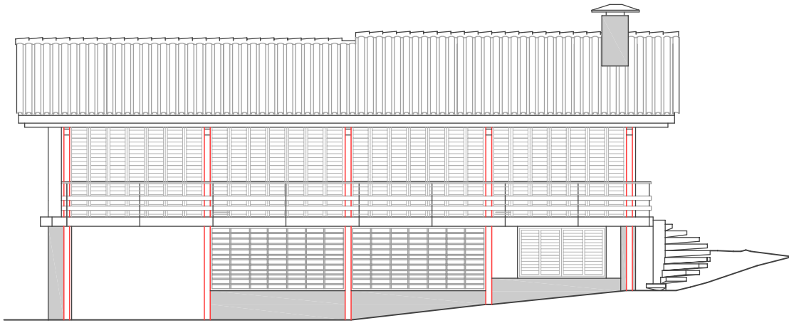
FAÇANA SUD. ESTAT INICIAL
