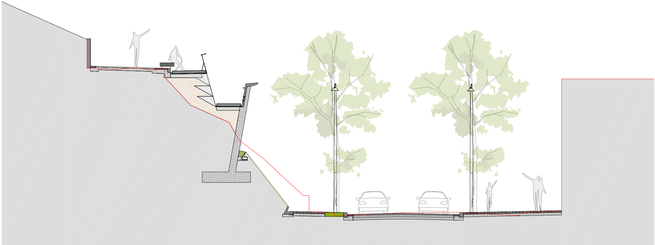
SECCIÓ TRANSVERSAL 0 1 2 3 4 5
