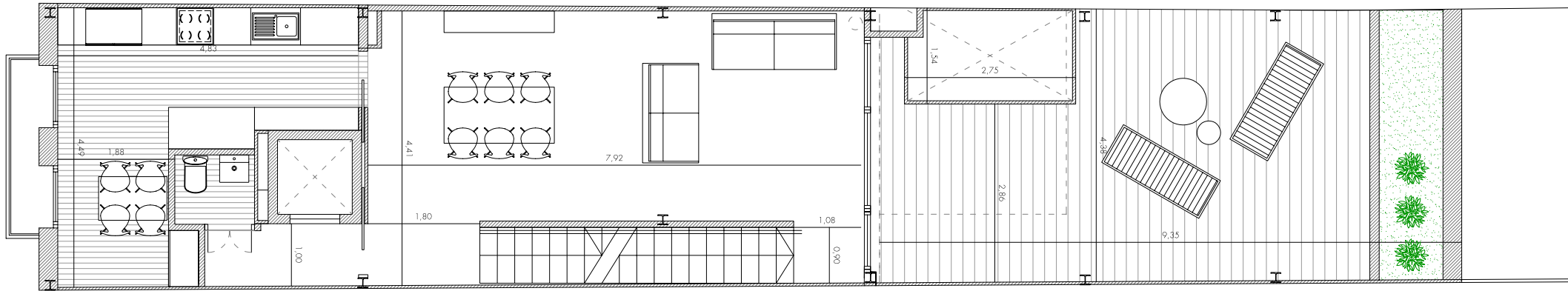
PLANTA PRIMERA
