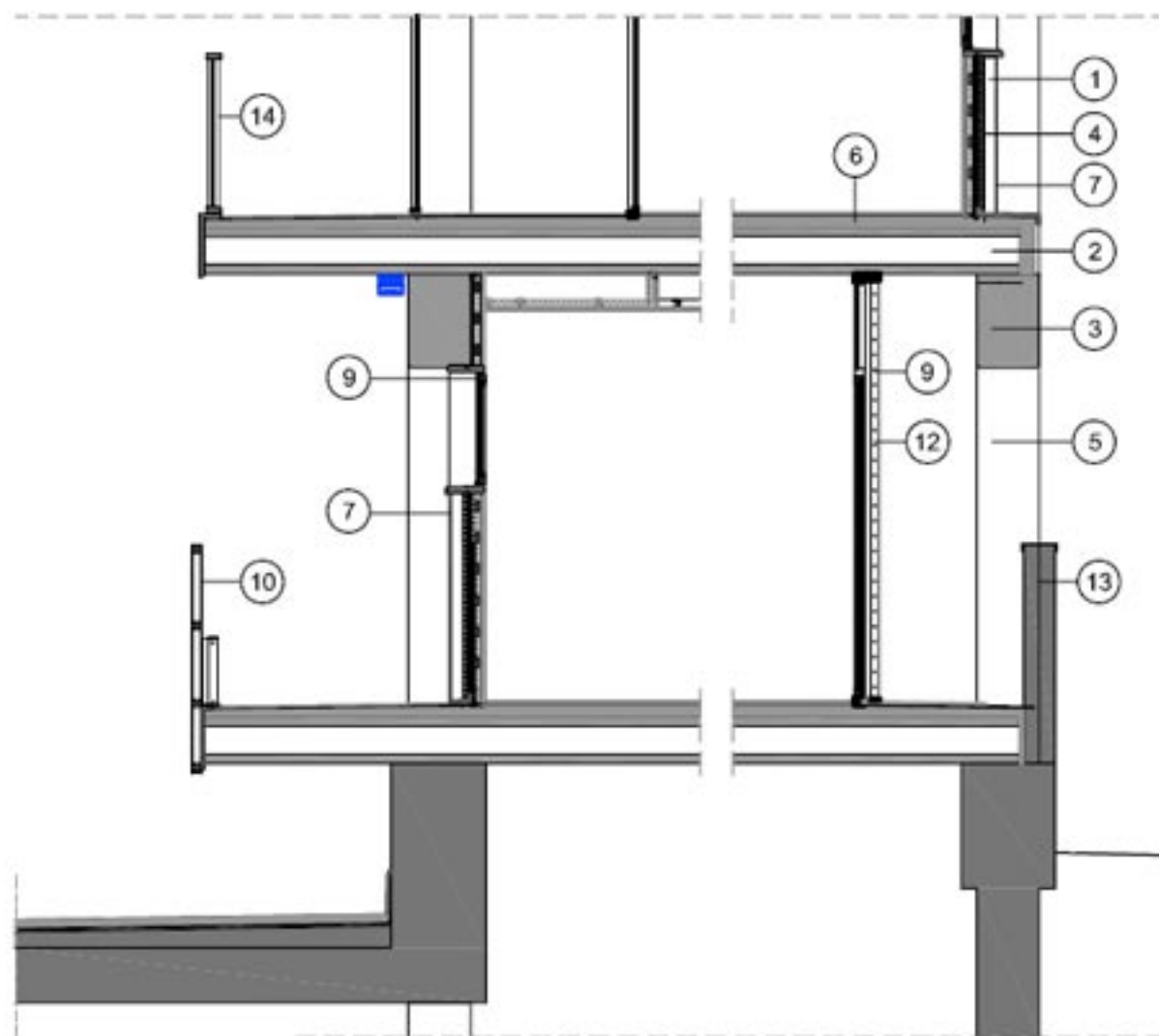
DETALL FAÇANA
