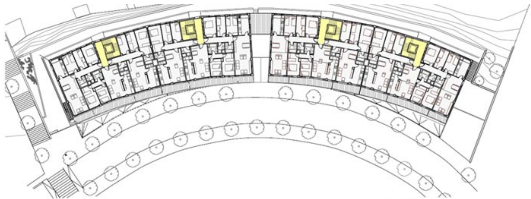
PLANTA TIPUS
