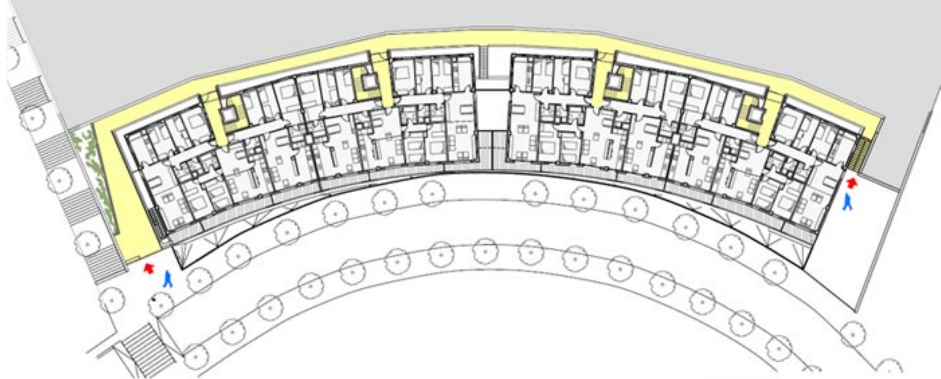
PLANTA PRIMERA
