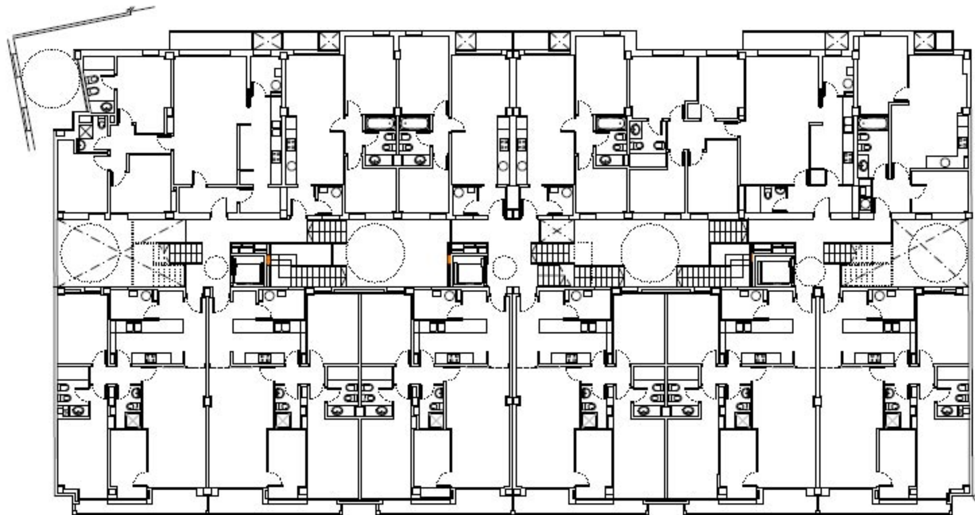
PLANTA TIPO
