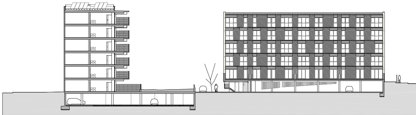
secció e-e'
