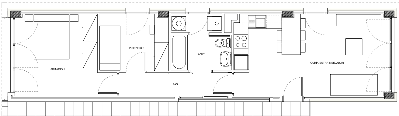
habitatge tipus 3 (2 habitacions)
