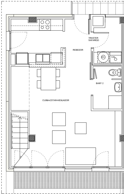
habitatge tipus 1 (duplex)
