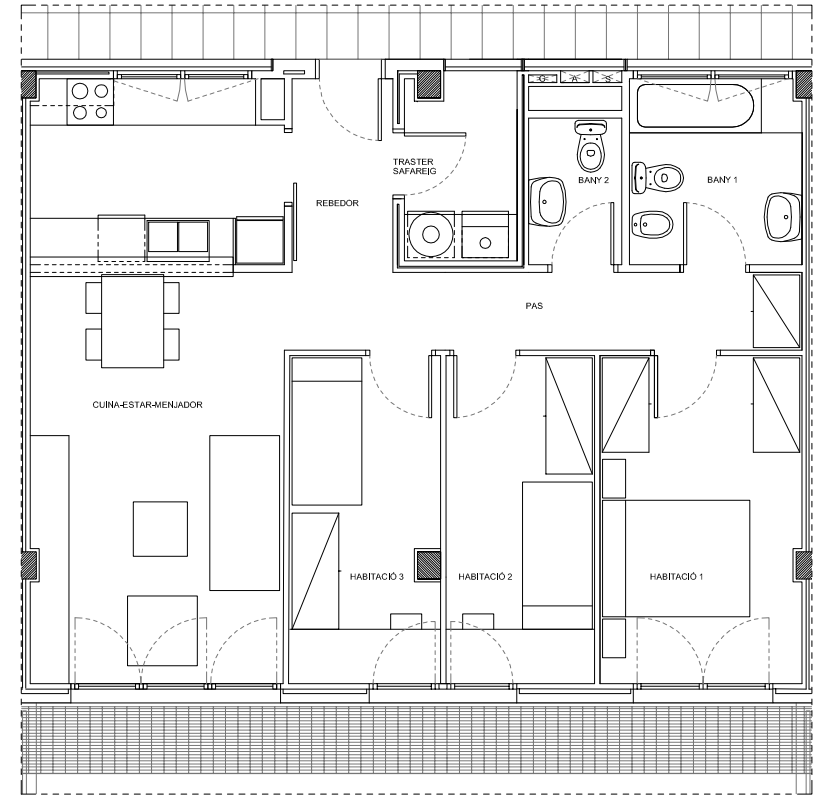
habitatge tipus 2 (3 habitacions)
