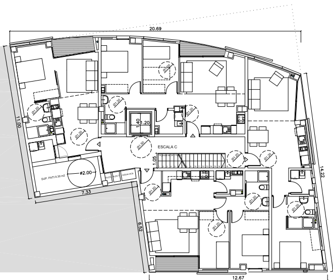
PLANTA TERCERA +233.50
