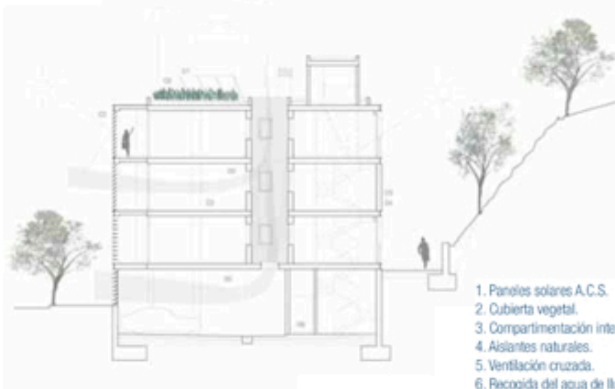
Sección tipo
