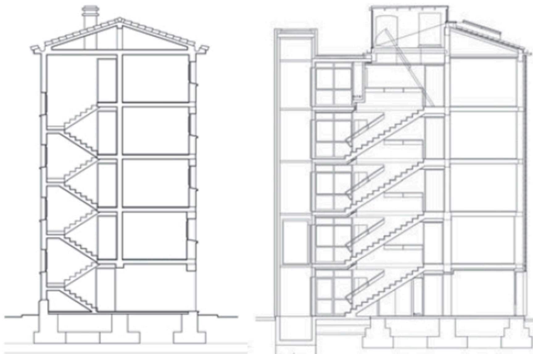
Secciones transversales.
