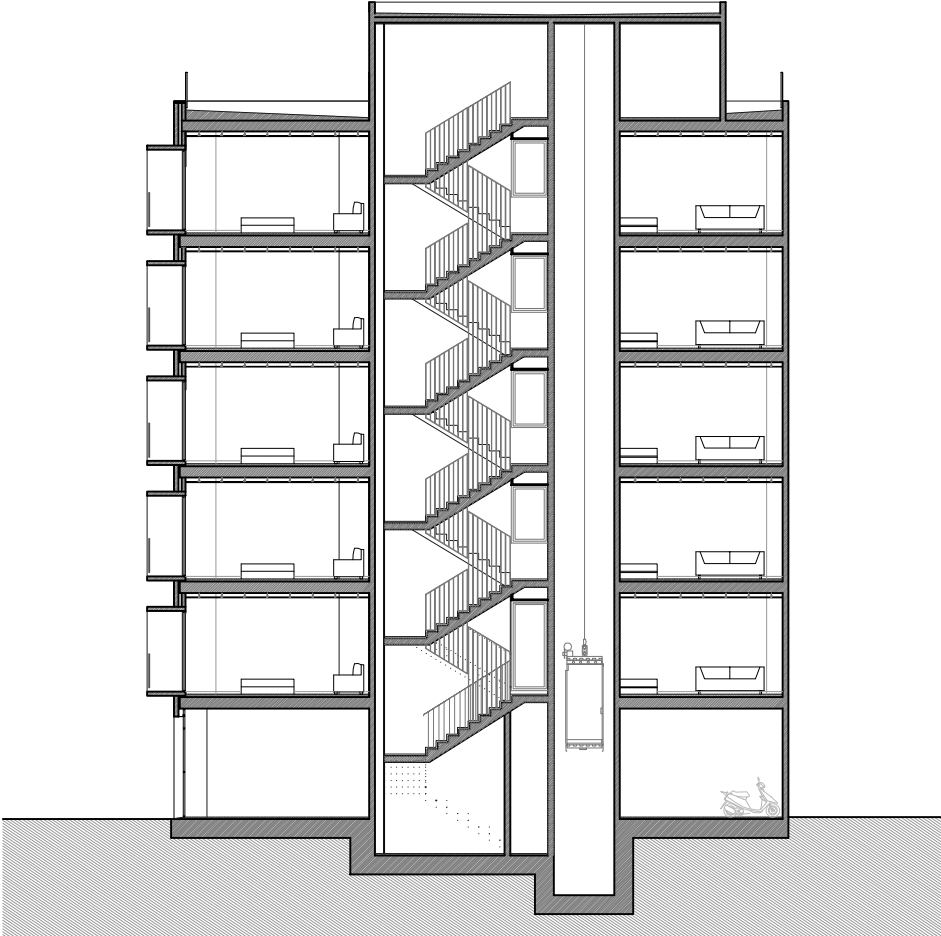
SECCIÓN LONGITUDINAL
