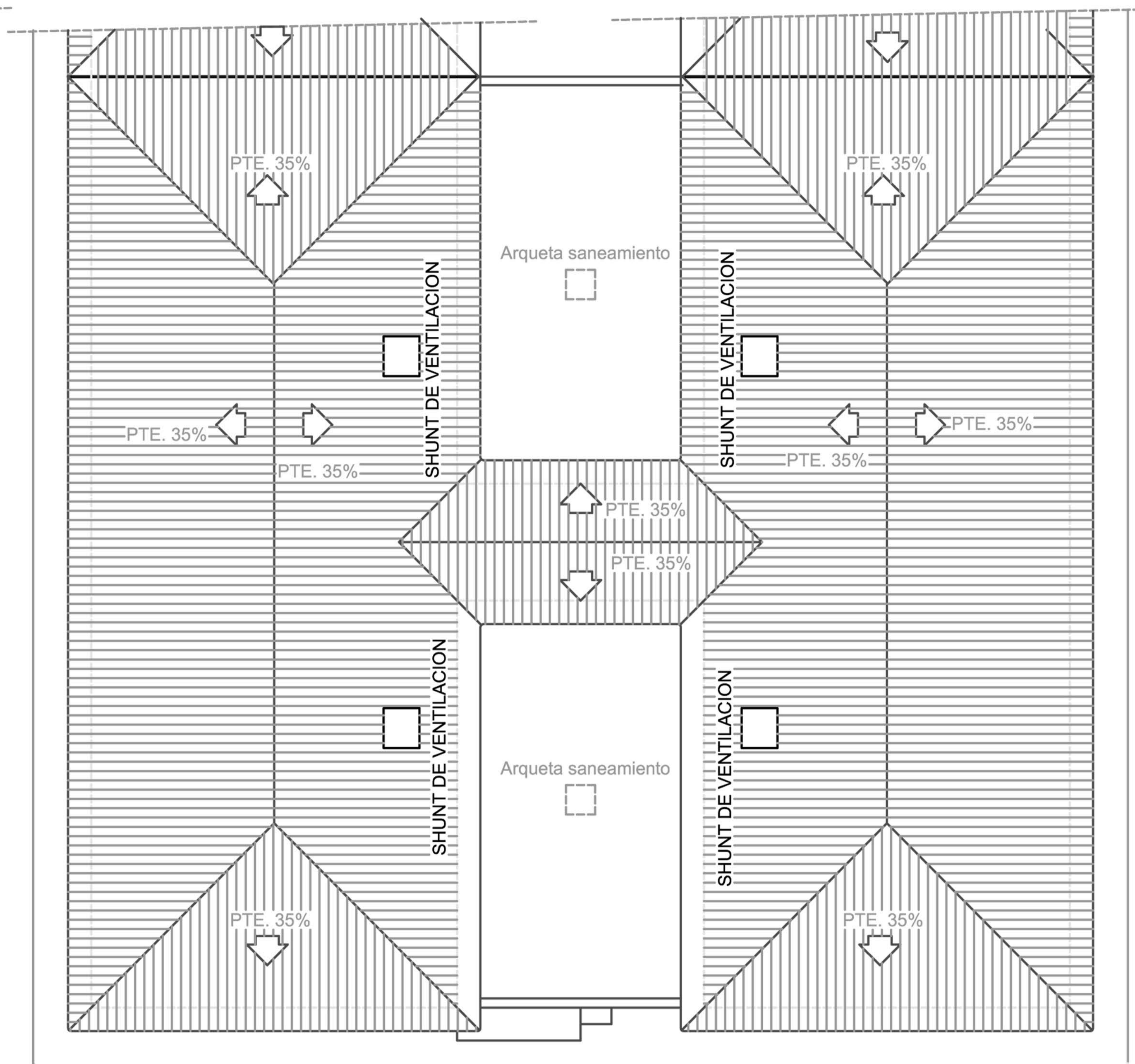
PLANTA CUBIERTA
