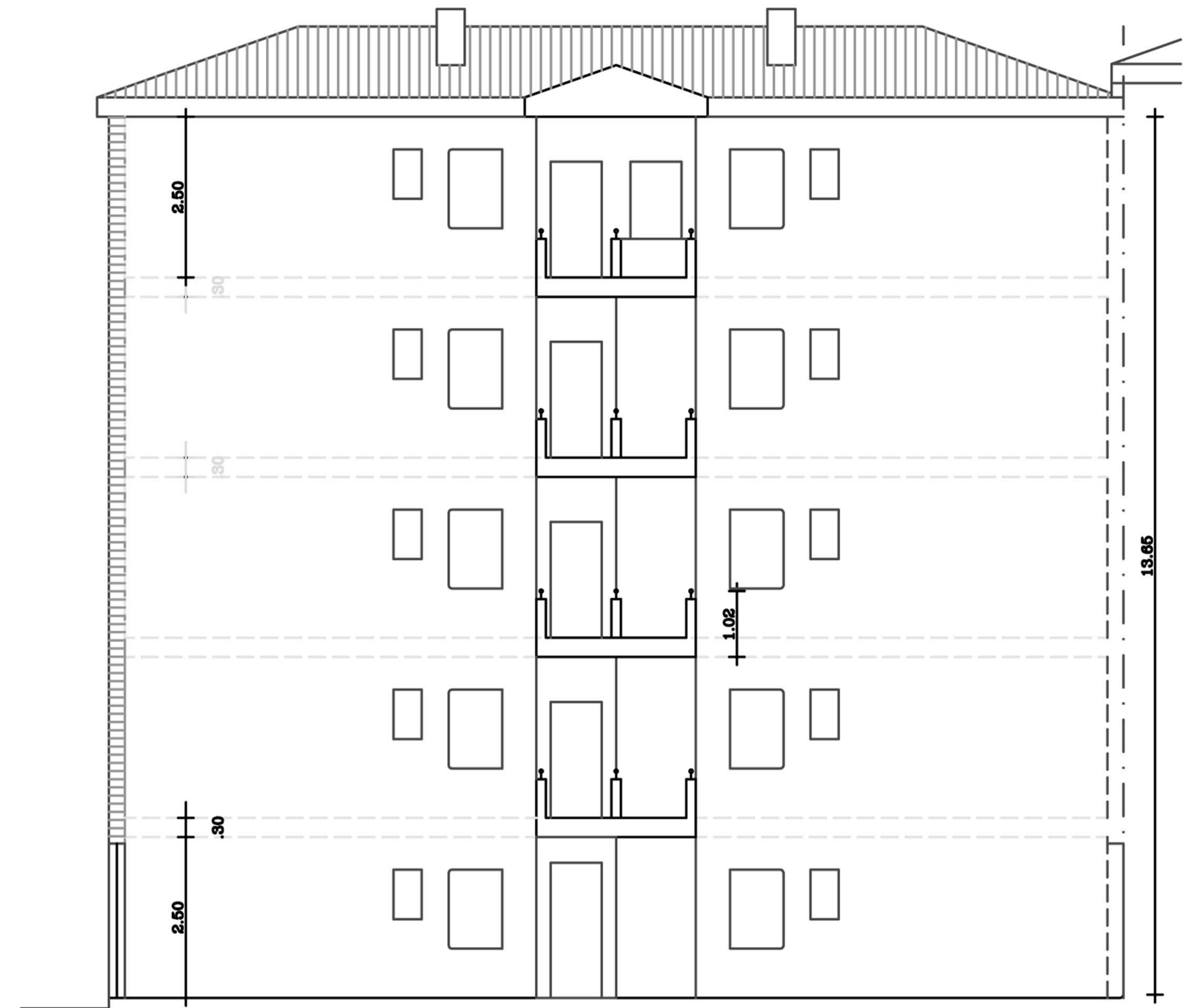
SECCION A-A
