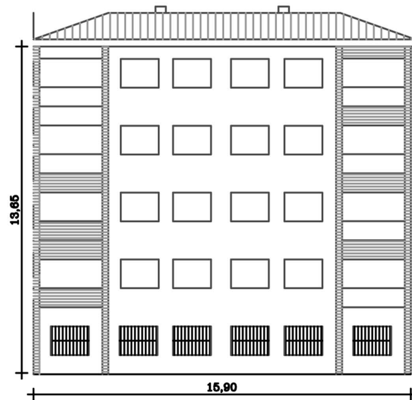
FACHADA LATERAL IZQUIERDA (E=1:100)
