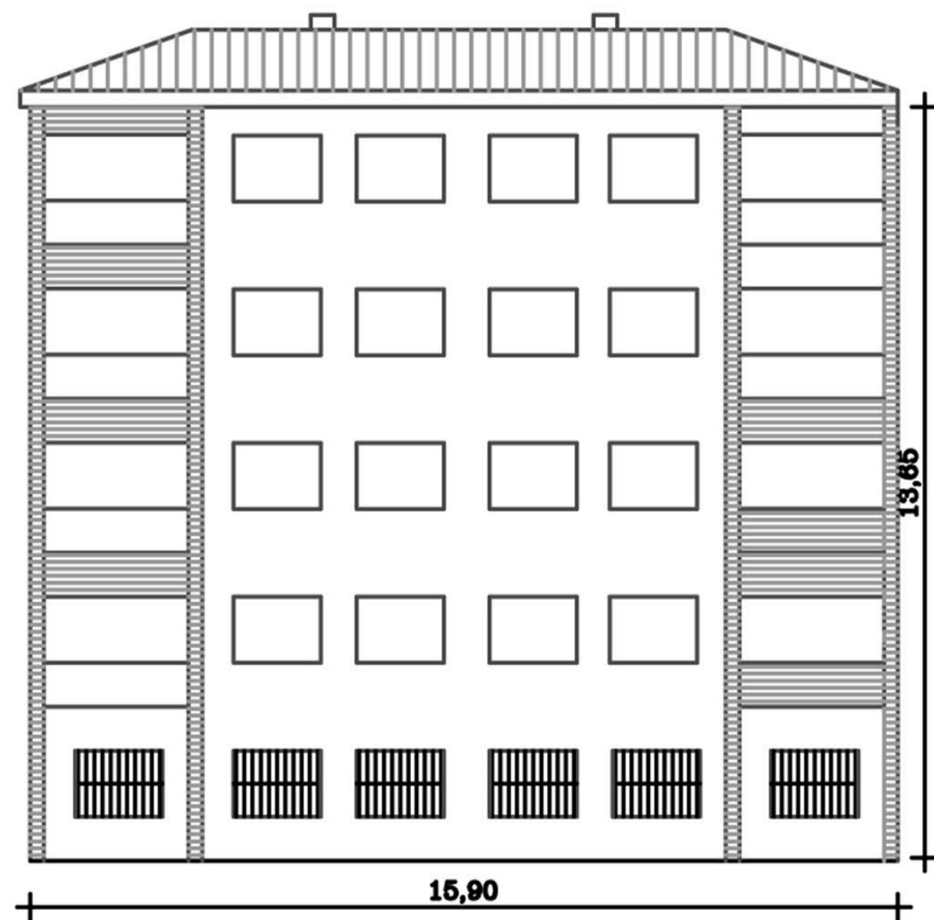
FACHADA LATERAL DERECHA (E=1:100)
