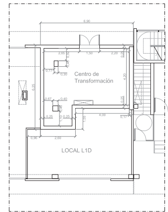
Variante de PLANTA BAJA en el BLOQUE 1.
