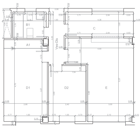
TIPO 1 (Variante A) SUPERFICIE ÚTIL = 55,83 m 2
