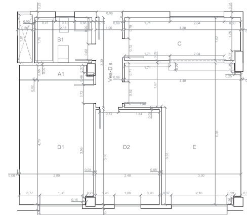
TIPO 1 (Variante C) SUPERFICIE ÚTIL = 55,63 m 2
