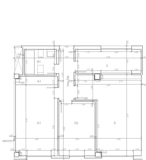
TIPO 1 (Variante D) SUPERFICIE ÚTIL = 55,77 m 2
