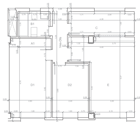
TIPO 1 (Variante B) SUPERFICIE ÚTIL = 55,80 m 2
