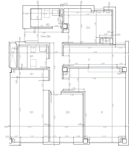
TIPO 3 SUPERFICIE ÚTIL = 68,85 m 2
