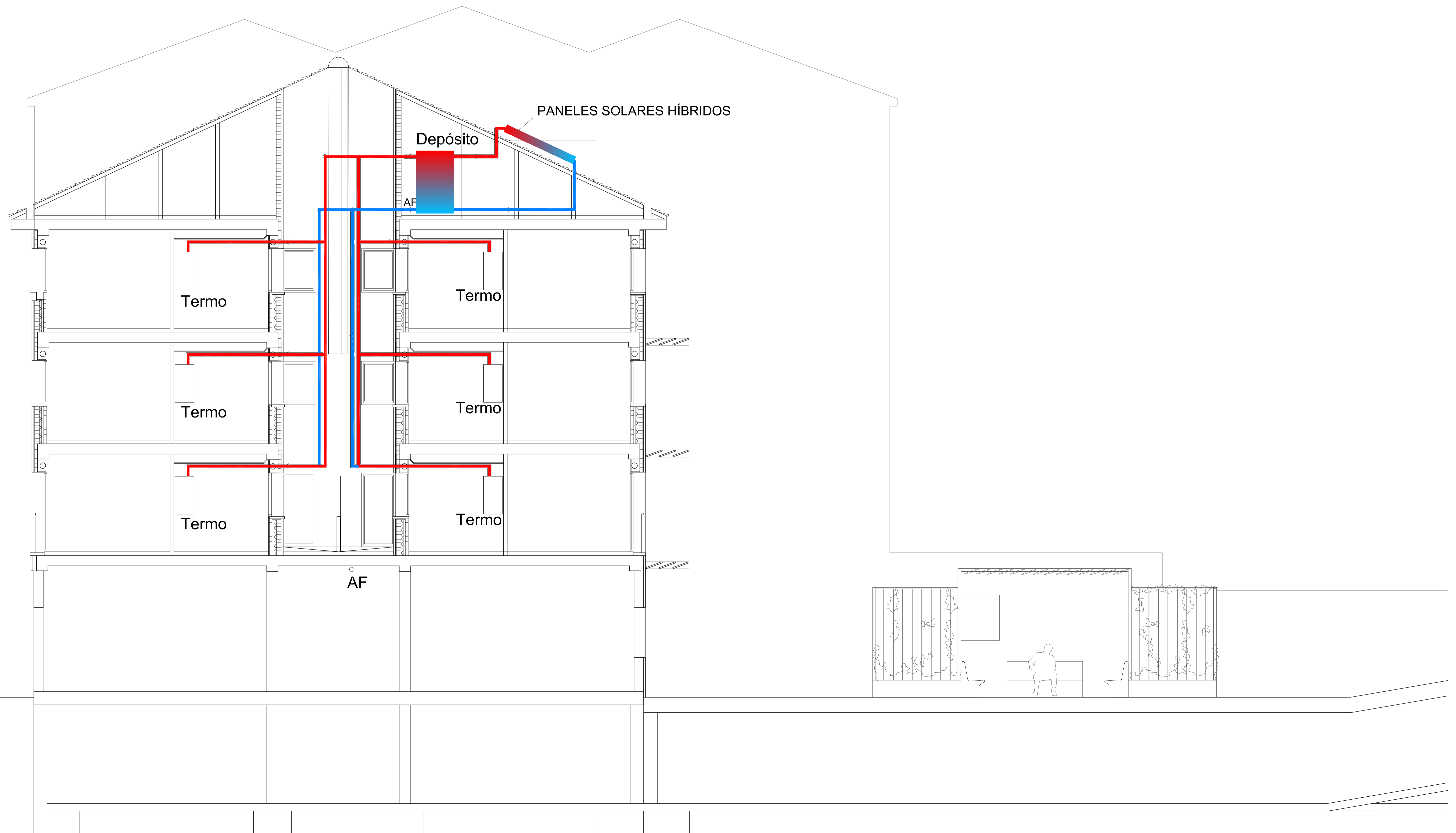
EDIFICIO A. SECCIÓN TRANSVERSAL POR PATIO. INSTALACIONES
