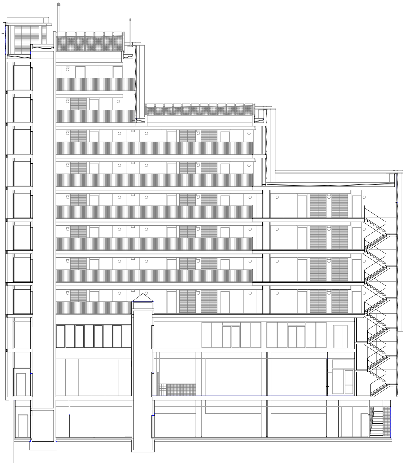
SECCION LONGITUDINAL
