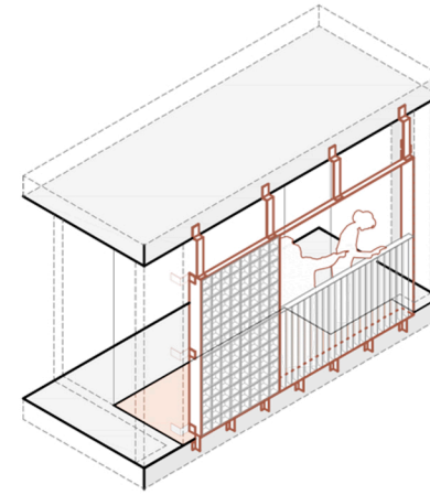
axonometria obertura tipus
