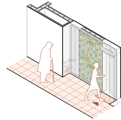
axonometria accés habitatges
