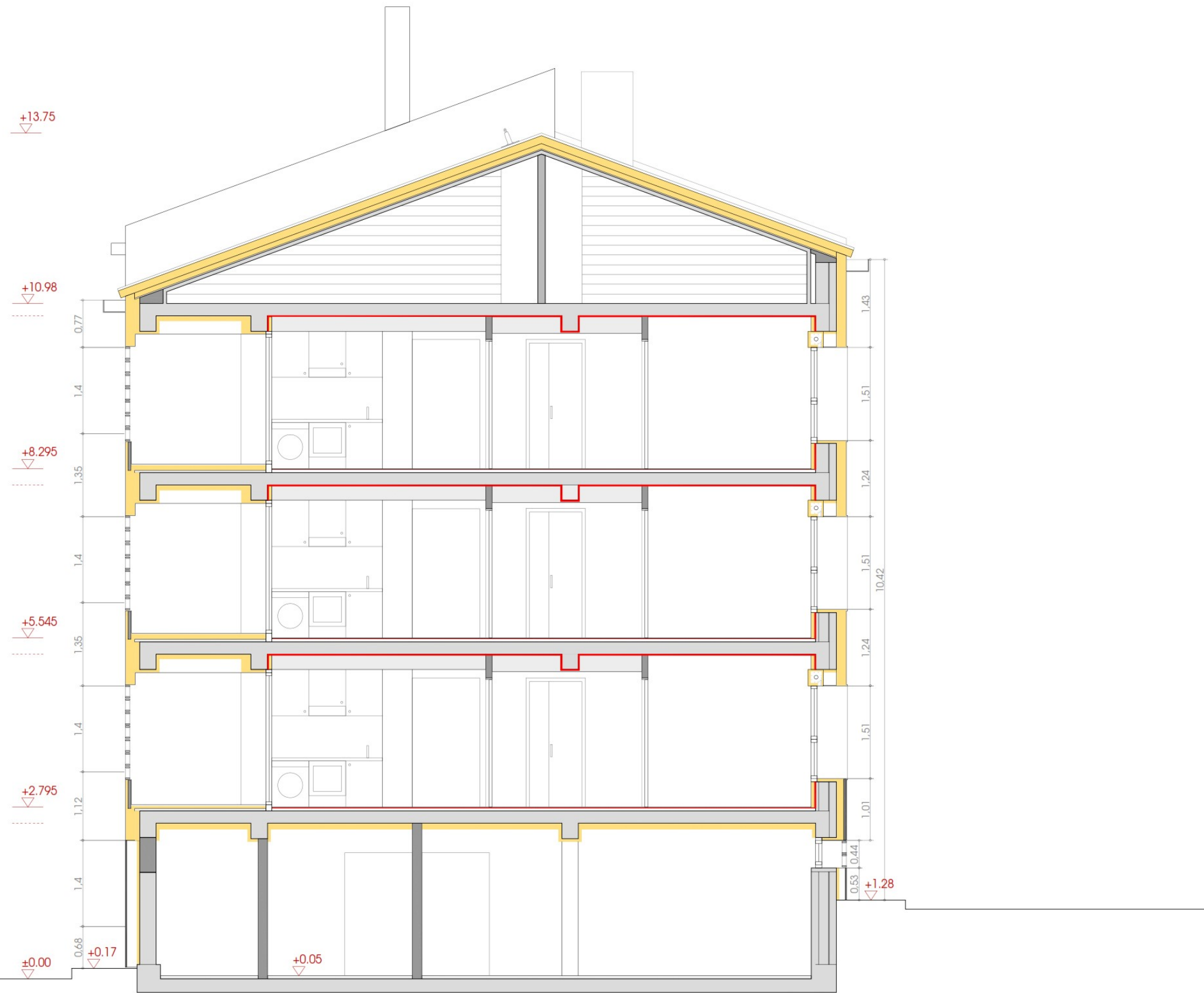
SECCIÓN S-2
