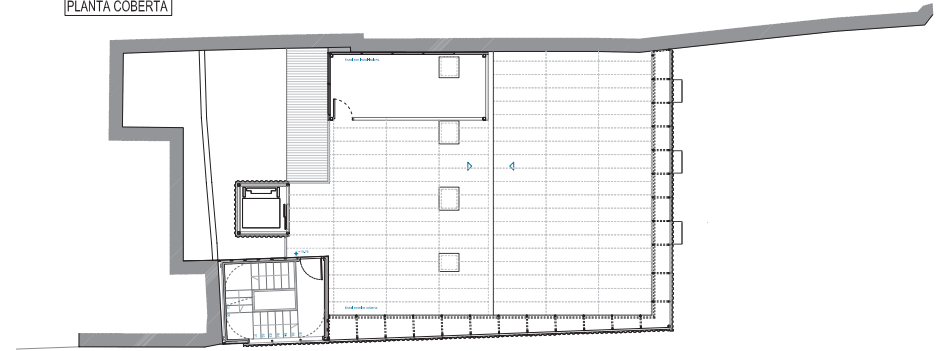
PLANTA COBERTA
