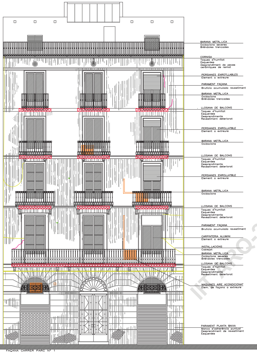
FAÇANA CARRER PARC Nº 1
