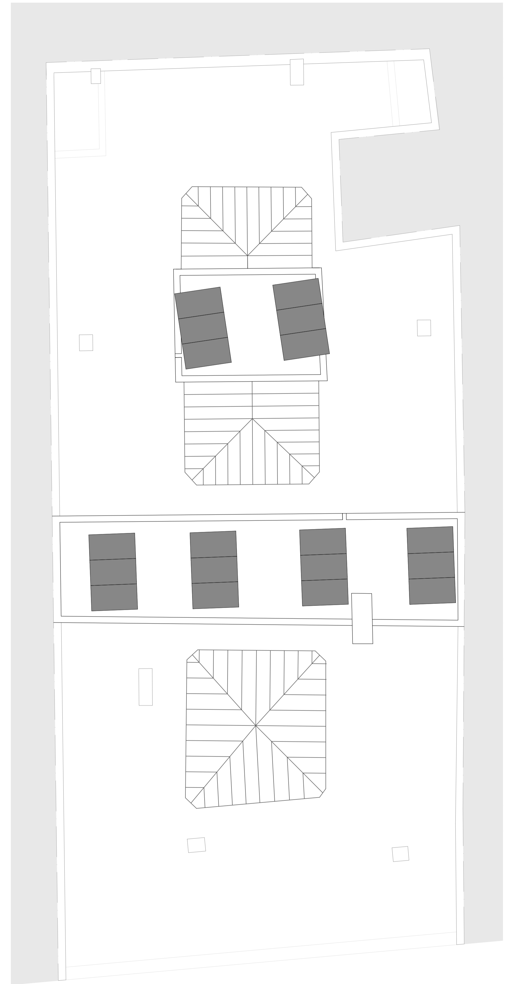
ESTADO REFORMADO PLANTA CUBIERTA
