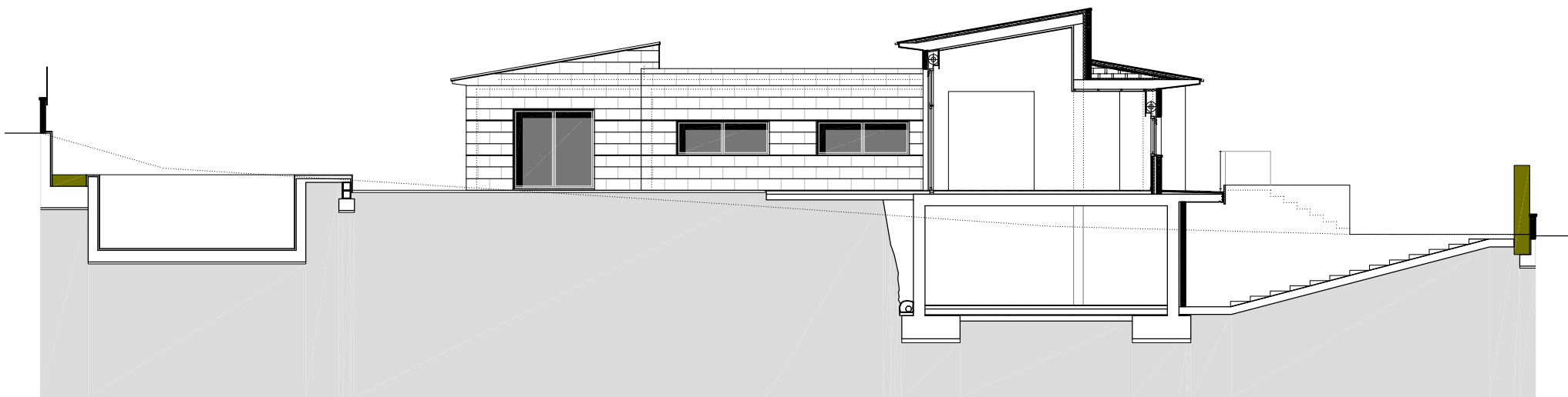
secció E
