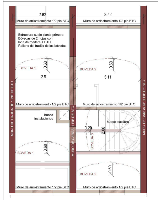
VIVIENDA 2. Planta 1ª. Esquema de estructura.
