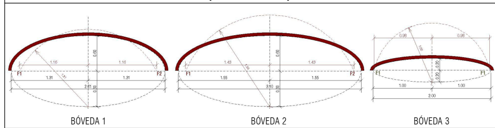
Replanteo bóvedas planta 1ª
