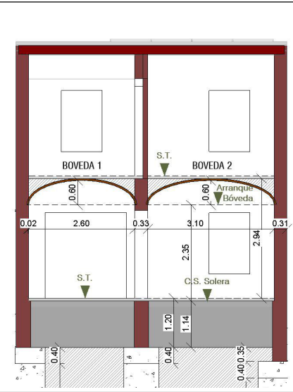
VIVIENDA 2. Sec transv. Esquema estructura.
