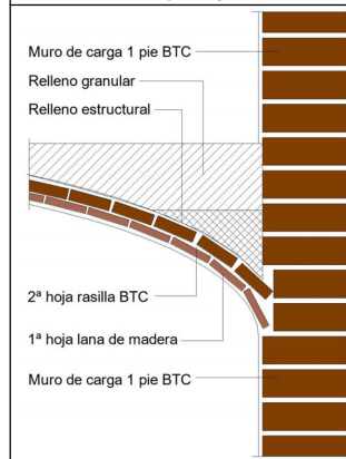
Bóveda forjado planta 1ª
