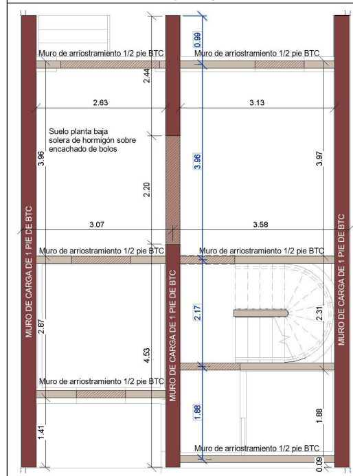
VIVIENDA 2. Planta Baja. Esquema de estructura.
