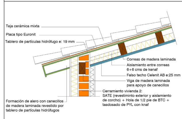
Alero fachada delantera
