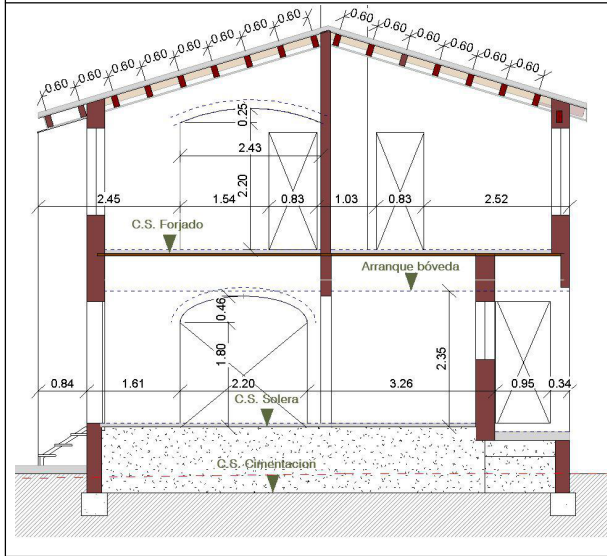
VIVIENDA 2. Sección longitudinal. Esquema de estructura.
