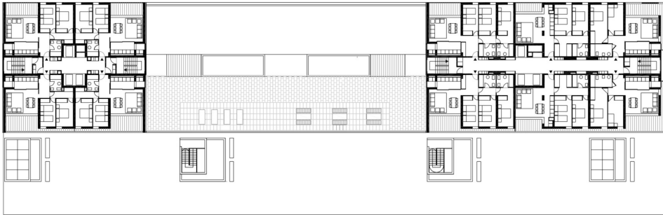
Planta cubierta 0 5 10m
