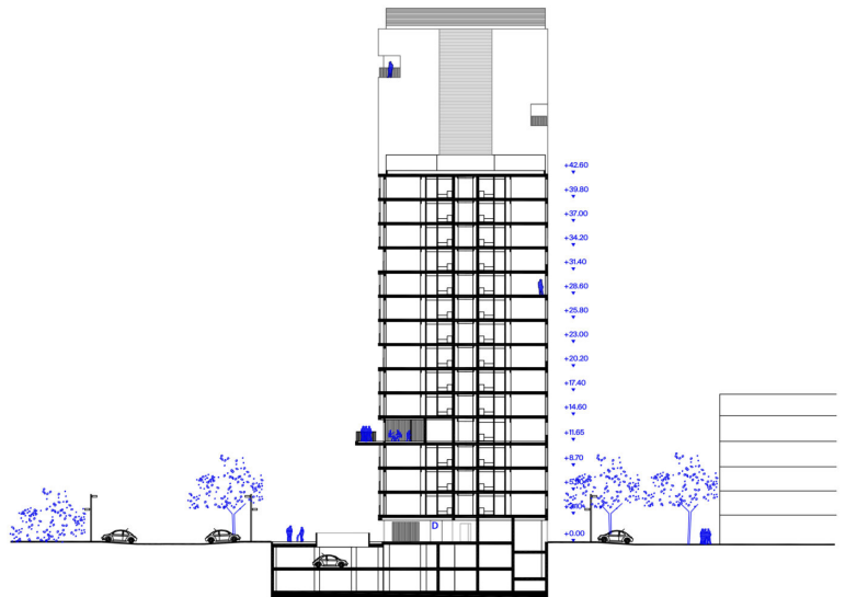
Sección 0 5 10m
