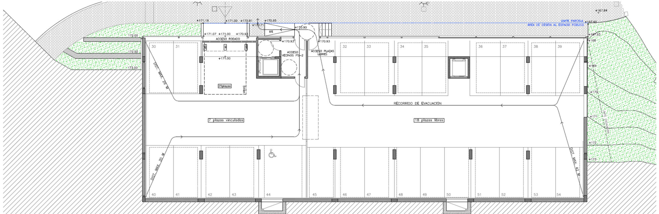
PLANTA SÓTANO -2 (+171.00)
