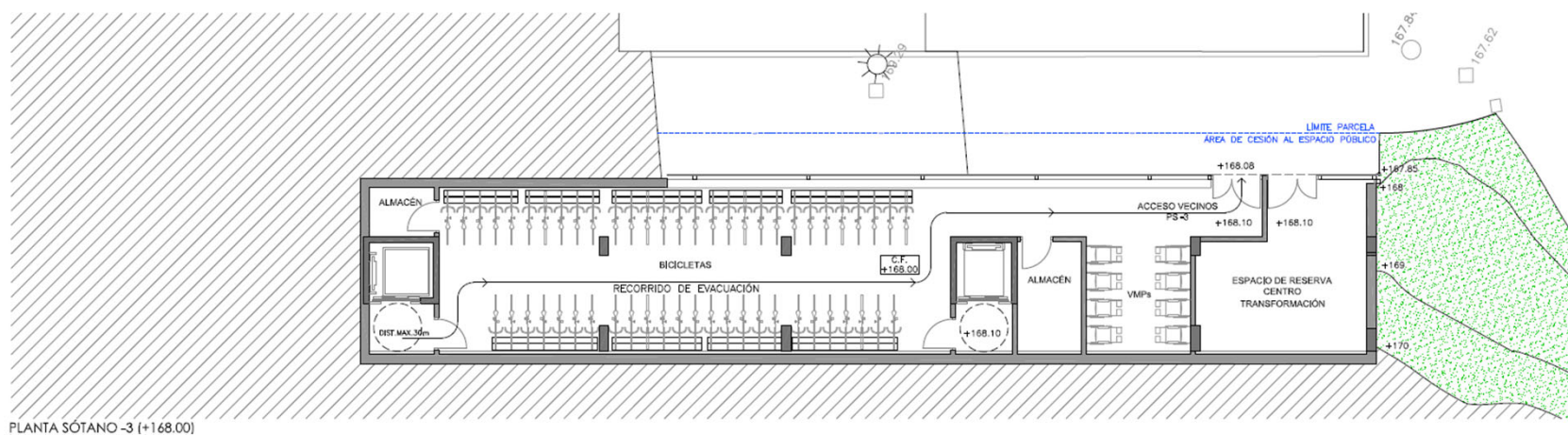
PLANTA SÓTANO -3 (+168.00)
