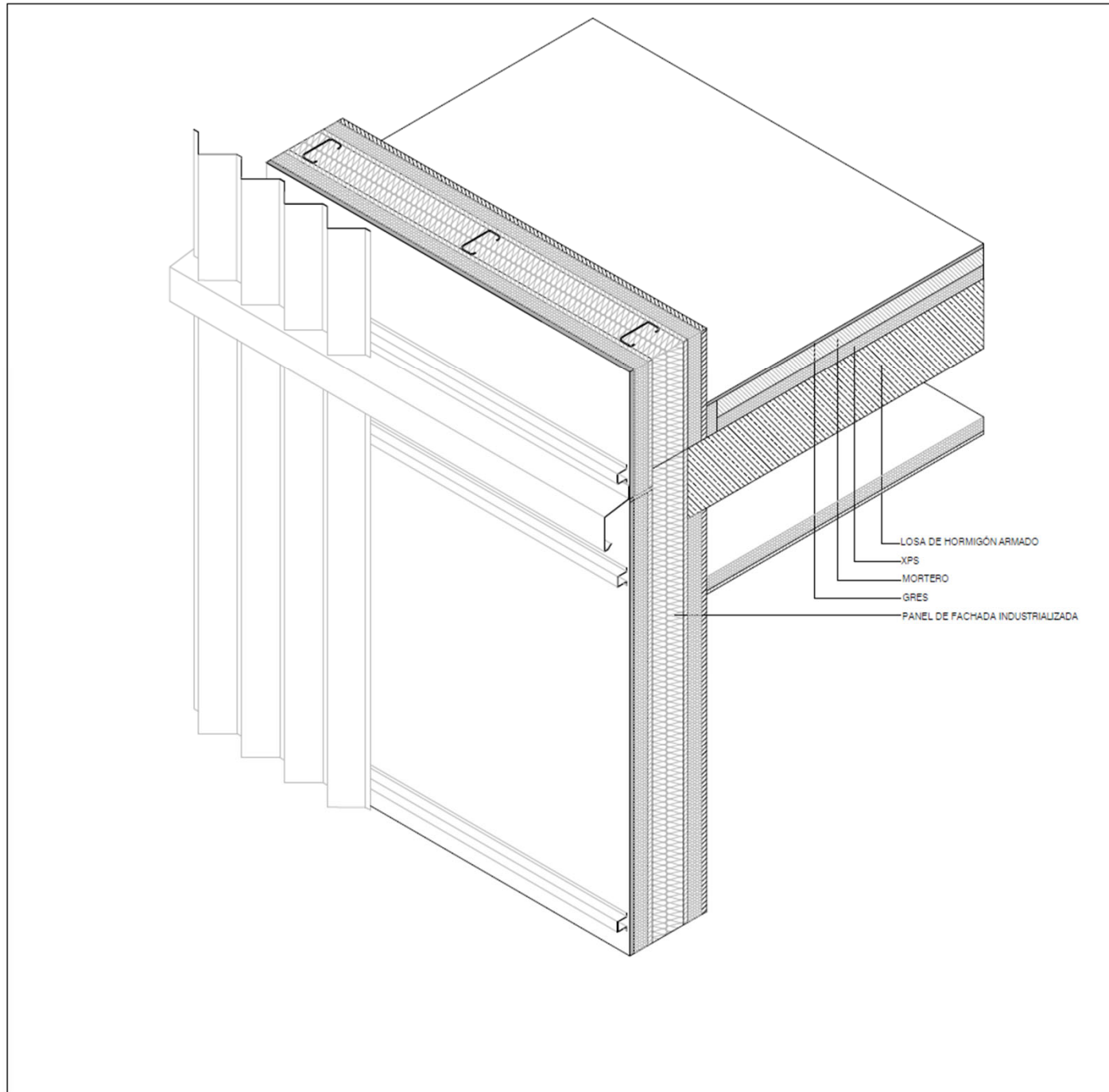
DETALLE ANCLAJE SUBESTRUCTURA Y PANEL COMPOSITE
