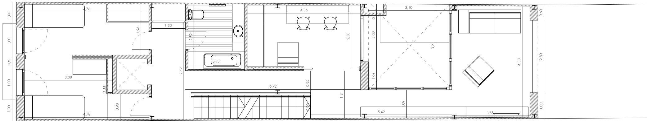
PLANTA SEGONA
