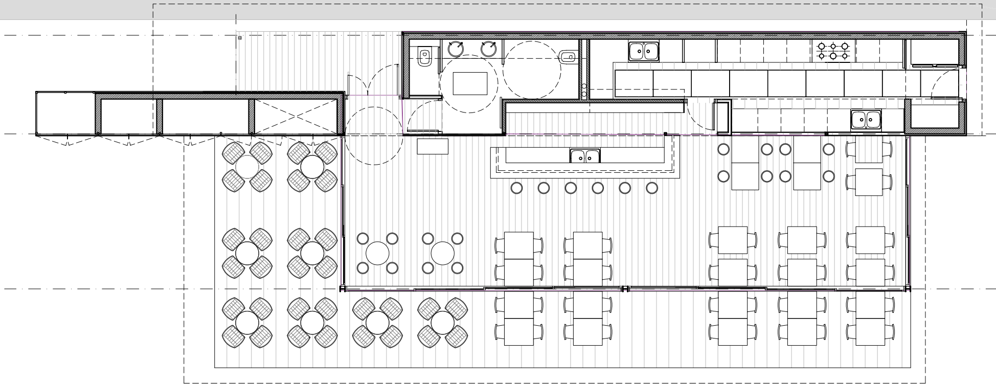
PLANTA 1/100
