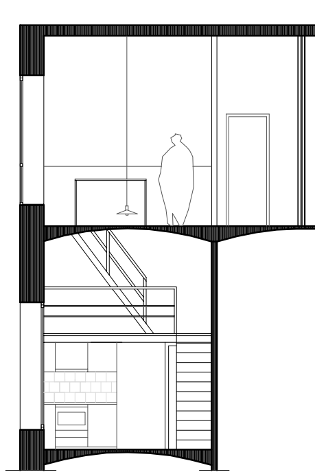
SECCIÓ TRANSVERSAL E. 1/100
