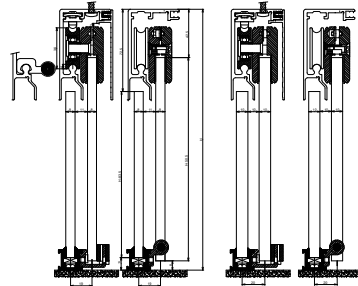
KLEIN ROLL GLASS 60(VB-10) A PORTES CORREDERES SECCIÓ VERTICAL
