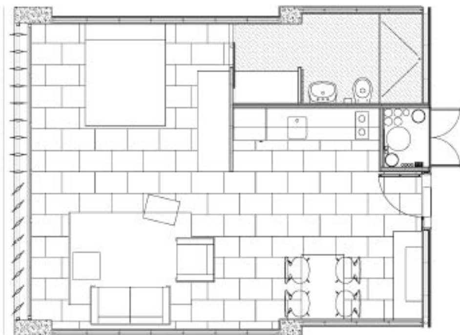
PLANTA TIPUS D'HABITATGE, 1/50
