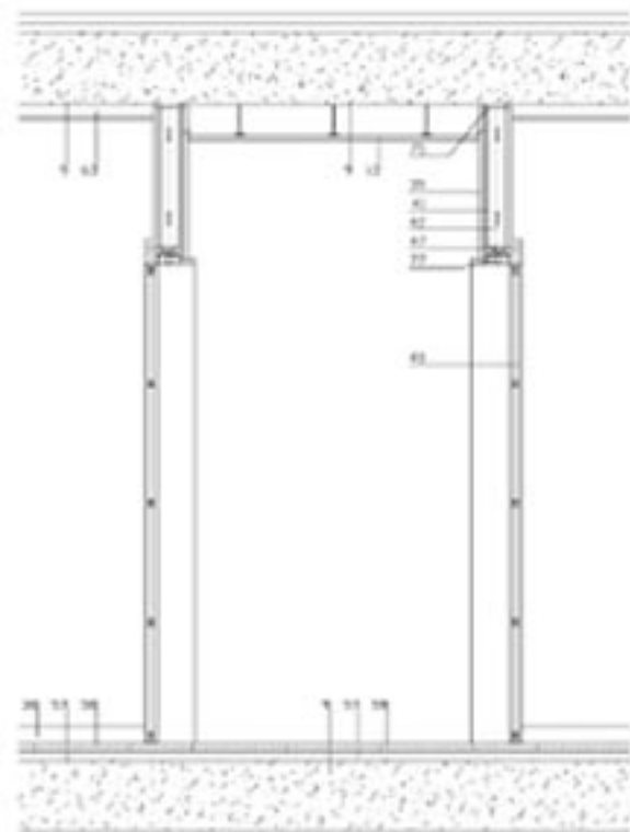
SECCIÓ CONSTRUCTIVA DEL PASSADÍS
