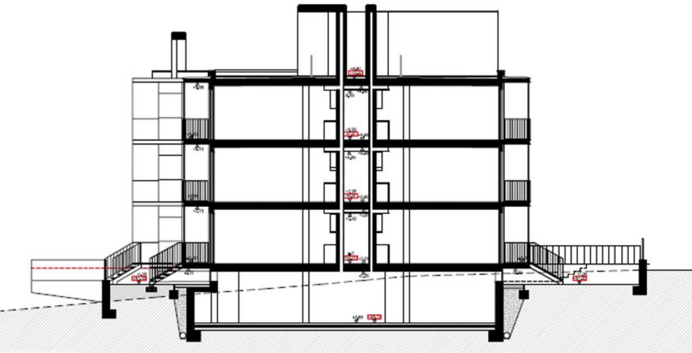
SECCIÓ A-A'
