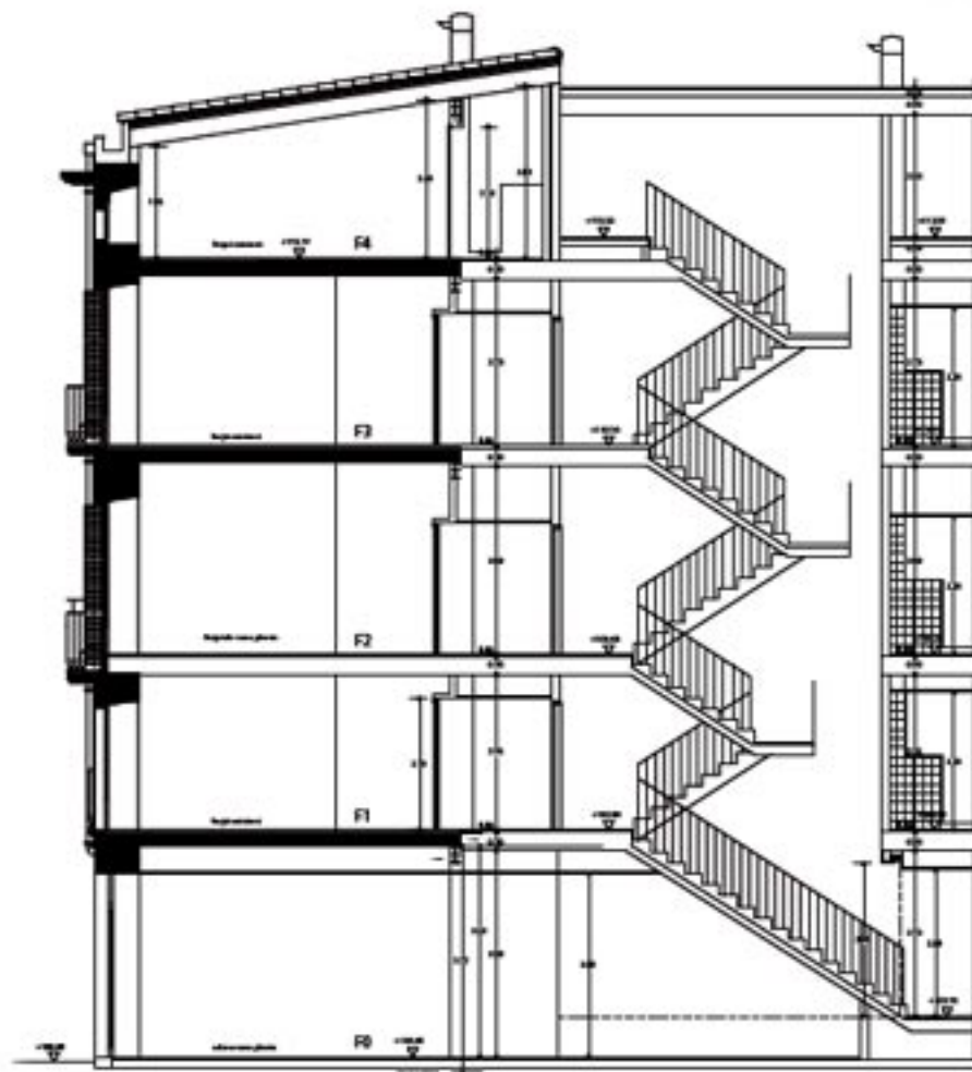
SECCIÓ LONGITUDINAL A-A
