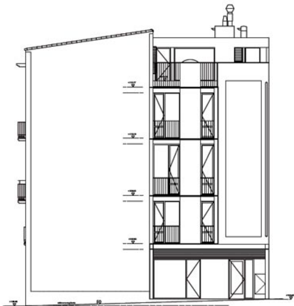
FAÇANA CARRER DEL CAMP D'URGELL
