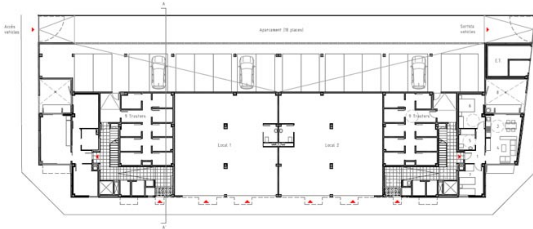
BLOC 1 Planta baixa 1/150 2 vivendes adaptades, 2 locals i aparcament
