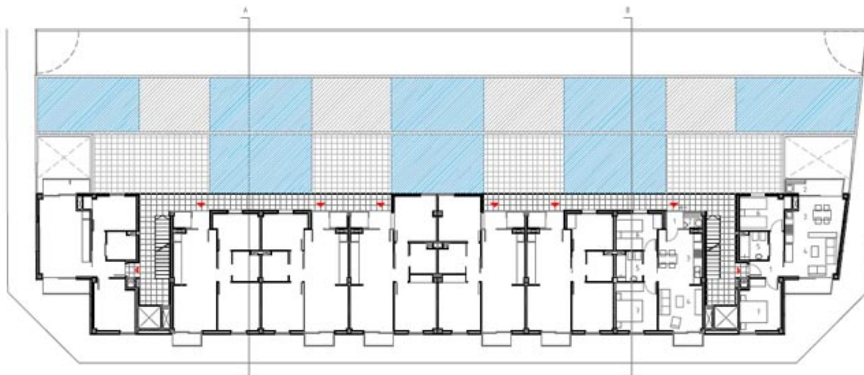
BLOC 1 Planta 1 i 2 1/150 8 vivendes per planta
