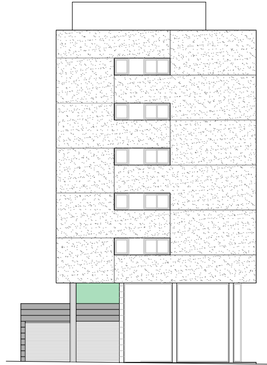
FAÇANA SUDOEST
