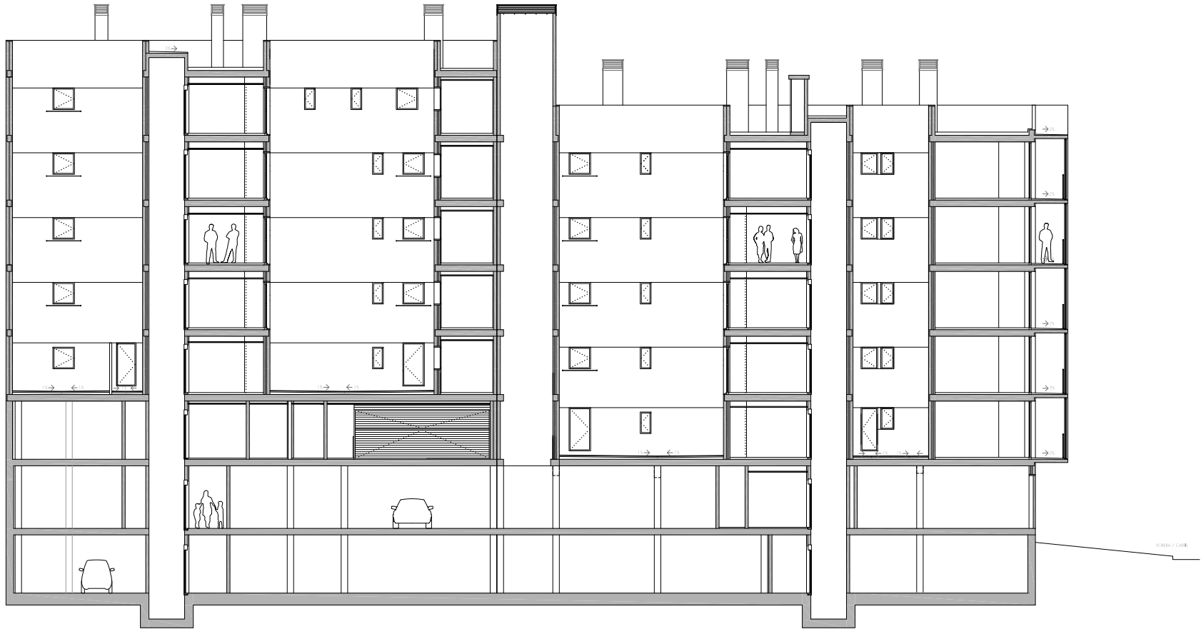
SECCIÓ LONGITUDINAL SL1
