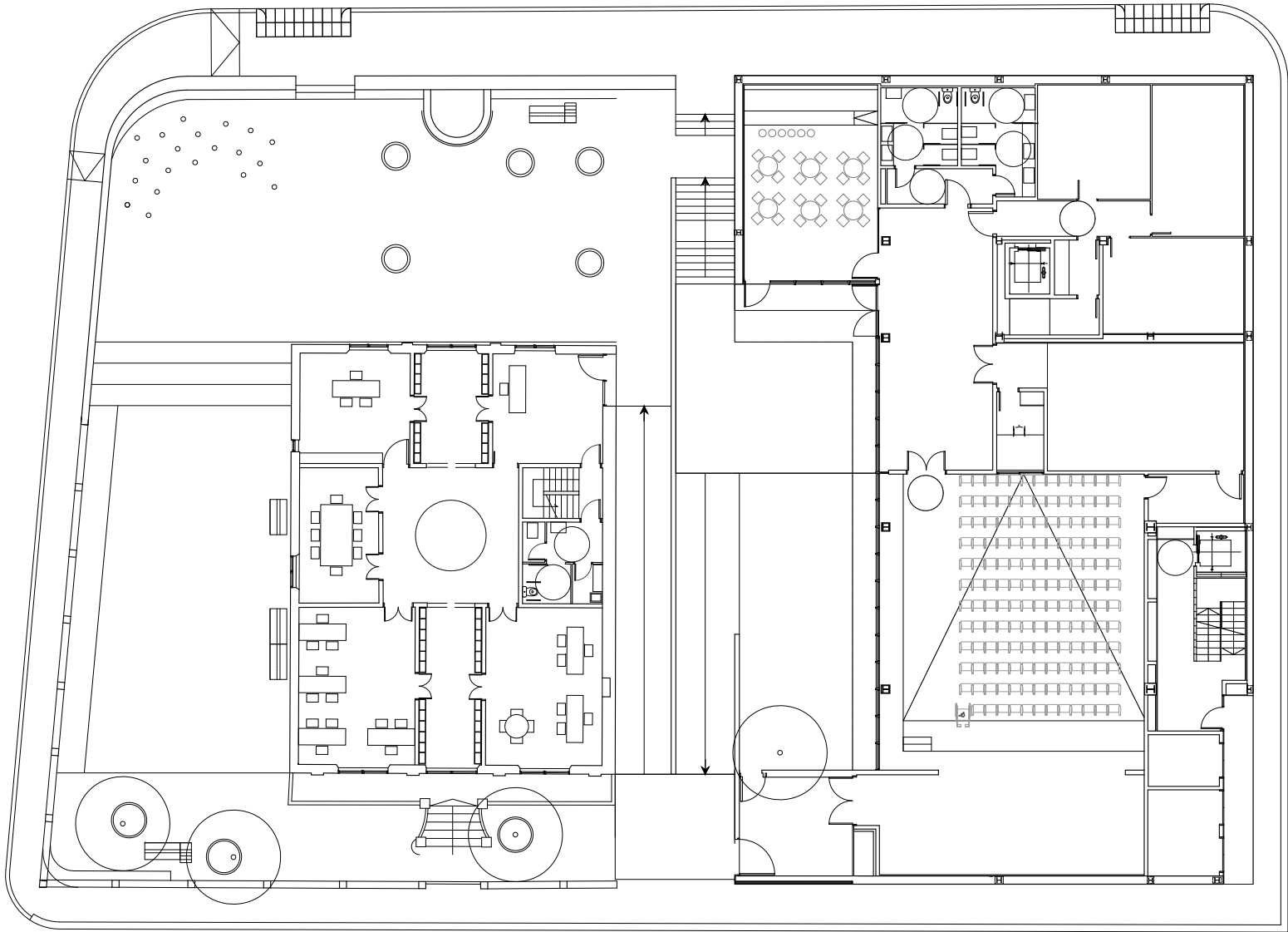
PLANTA SOTERRANI
